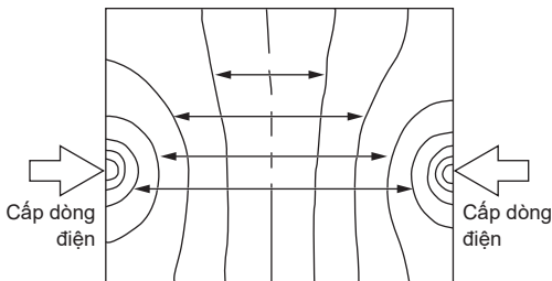
Hình 1: Các đường đẳng thế trên một tấm kim loại, cho thấy phân phối dòng điện ở các khoảng 50 \mu\text{V} khi dòng điện 1 A được cấp cho từ điểm cuối của tấm ( R300 \times D370 \times t0,4 )
